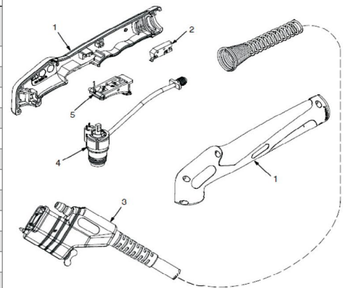
XT60 Torch
