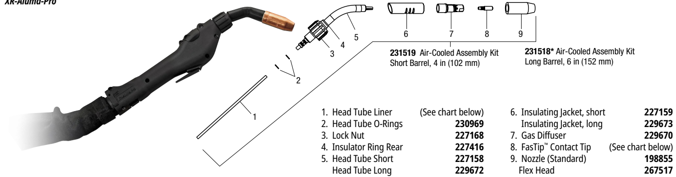
XR-Aluma-Pro
